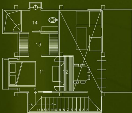
PLANTA ARQUITECTONICA 0+5.56 ESCALA 1:75
