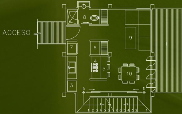
PLANTA ARQUITECTONICA 0+2.78 ESCALA 1:75
