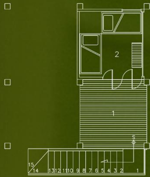
PLANTA ARQUITECTONICA 0+00 ESCALA 1:75
